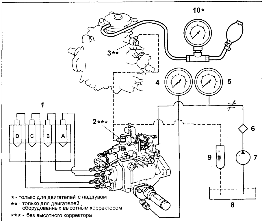
Схема стенда. 1- форсунки, 2 и 3 - возвратный топливопровод, 4 и 5 - манометры давления топлива, 6- фильтр стенда, 7 - насос стенда, 8- топливный бак стенда, 9 расходомер стенда, 10 - приспособление.
