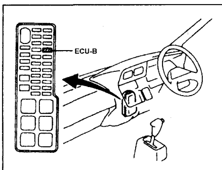
Hi-Ace (1KZ-TE).
