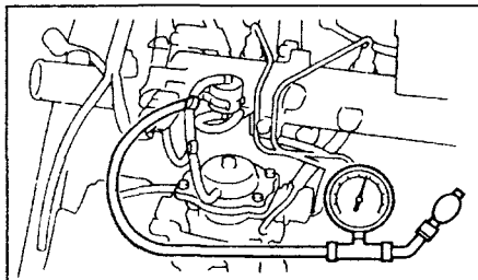
Двигатель 1KZ-T.
