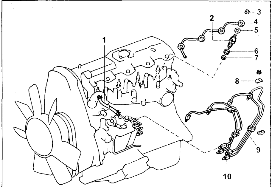
Снятие форсунок (серия L). 1 - топливный шланг, 2 - форсунка М.З. 64 Н·м, 3 - гайка М.З. 29 Н·м, 4 - дренажная трубка, 5, 7 - прокладка, 6 - уплотняющая шайба, 8 - зажим, 9 - трубка высокого давления, 10 - гайки трубок М.З. 25 Н·м.
