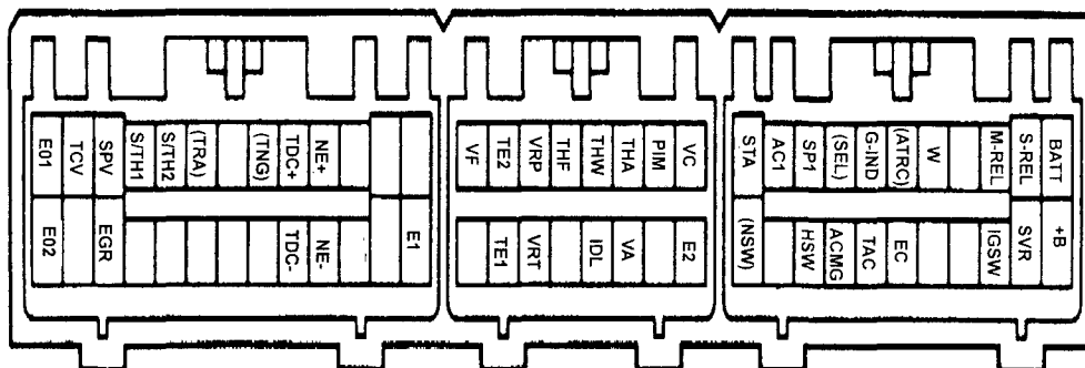
Разъем электронного блока управления двигателя 2L-TE (Mark II с августа 1995)
