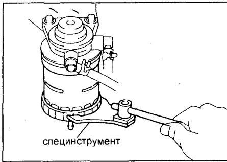
Б. Клещами отверните датчик наличия воды.
