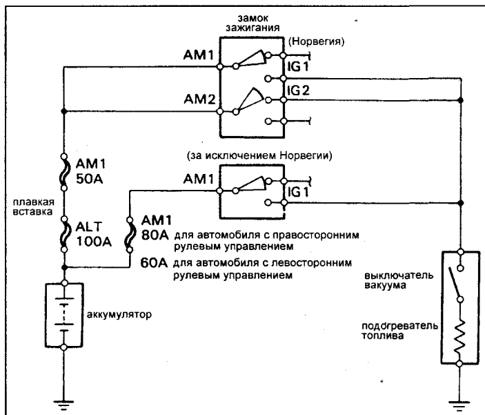
Схема системы подогрева топлива (HiAce для Европы).
