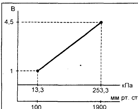
Зависимость напряжения от давления (KZN165).
