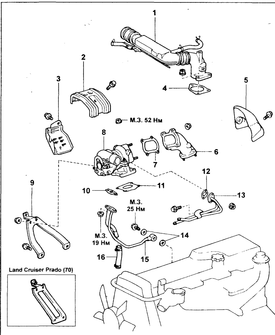
Двигатель 2L-T. 1 - впускной воздуховод, 2 - тепловой экран №1, 3 - тепловой экран №2, 4 - прокладка, 5 - тепловой экран №3, 6 - выпускной патрубков, 7, 10, 11, 12, 14 - прокладка, 8 - турбокомпрессор, 9 - опора выпускного коллектора (HiLux), 13 - трубки системы охлаждения турбокомпрессора, 15 - трубка подачи масла, 16 - шланг слива масла.
