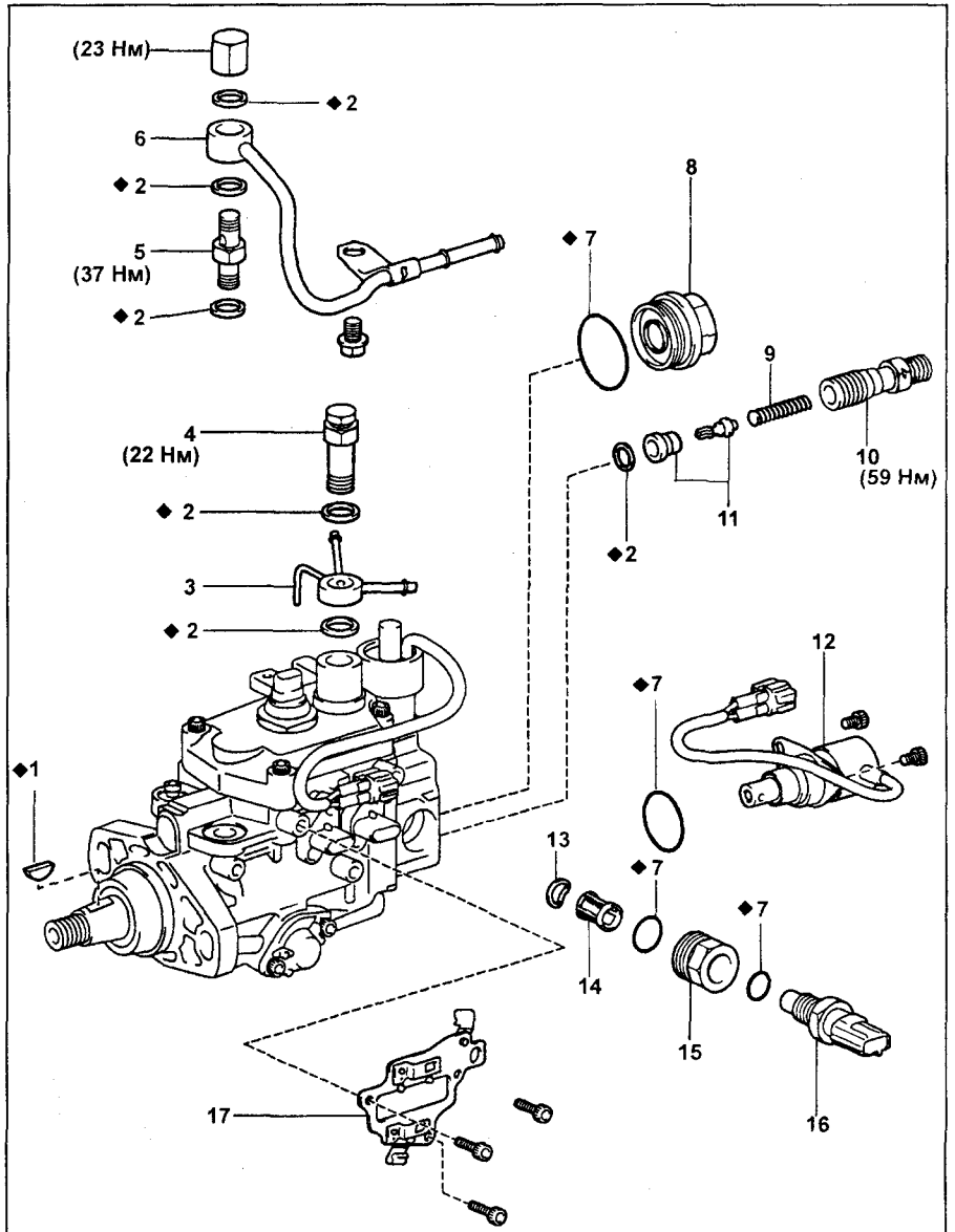
ТНВД. 1 - шпонка, 2 - прокладка, 3 - возвратный топливопровод, 4 - редукционный клапан, 5 - штуцер подачи топлива, 6 - трубка подачи топлива, 7 - уплотнительное кольцо, 8 - пробка распределительной головки №1, 9 - пружина, 10 - штуцер нагнетательного клапана, 11 - нагнетательный клапан, 12 - электромагнитный клапан регулировки угла опережения впрыска, 13 - фигурная шайба, 14 - сетчатый фильтр, 15 - пробка распределительной головки №2, 16 - датчик температуры топлива, 17 - кронштейн.
