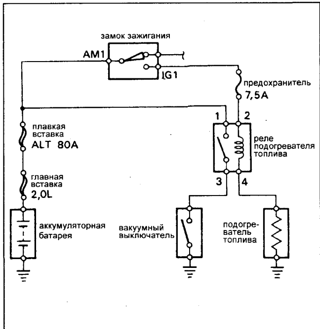
Схема системы подогрева топлива (Hilux).
