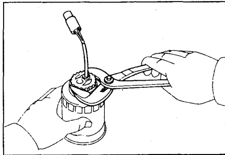
В. Переставьте датчик на новый топливный фильтр.
