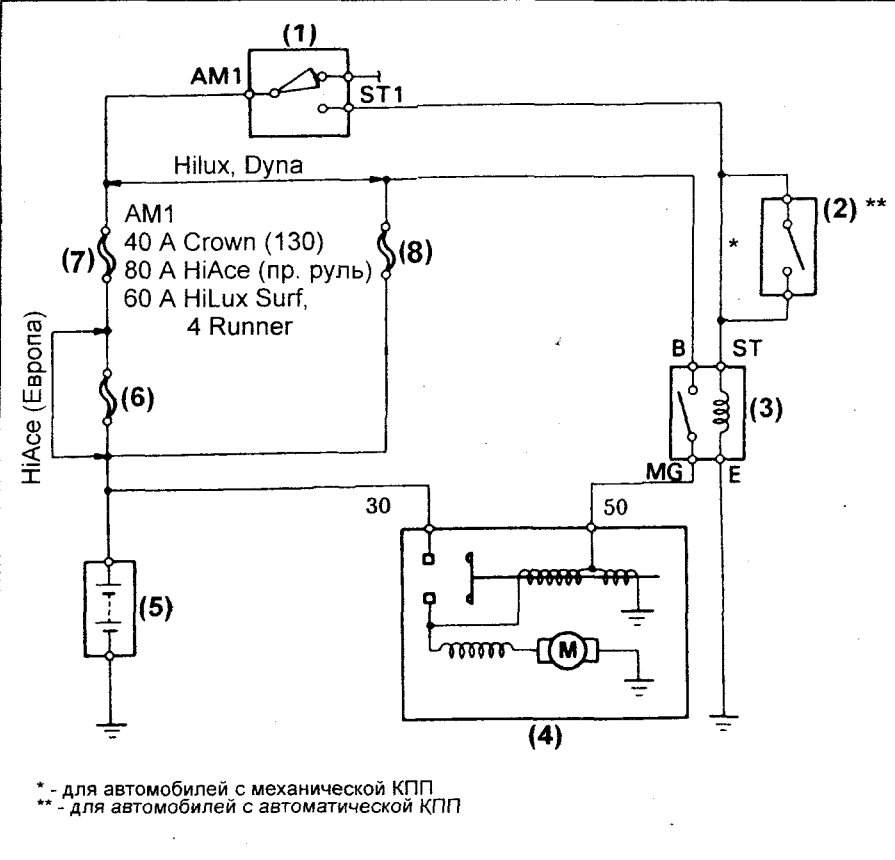
Электрическая схема системы пуска (двигатели серии L). 1 - замок зажигания, 2 - выключатель запрещения запуска двигателя, 3 - реле стартера, 4 - стартер, 5 - аккумулятор, 6, 7, 8 - плавкая вставка 80 - 100 А
