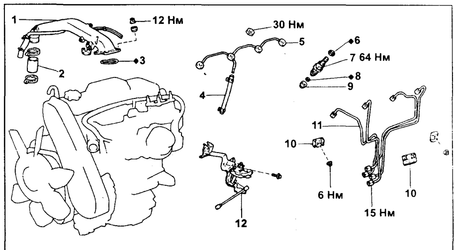
Снятие форсунок (серия KZ). 1 - впускной воздуховод, 2 - шланг, 3 - прокладка, 4 - шланг возврата топлива, 5 - дренажная трубка, 6 - уплотнительная шайба, 7 - форсунка, 8 - уплотнительная шайба, 9 - седло форсунки, 10 - зажим, 11 - топливная трубка высокого давления, 12 - кронштейн и тяга привода рычага ТНВД.
