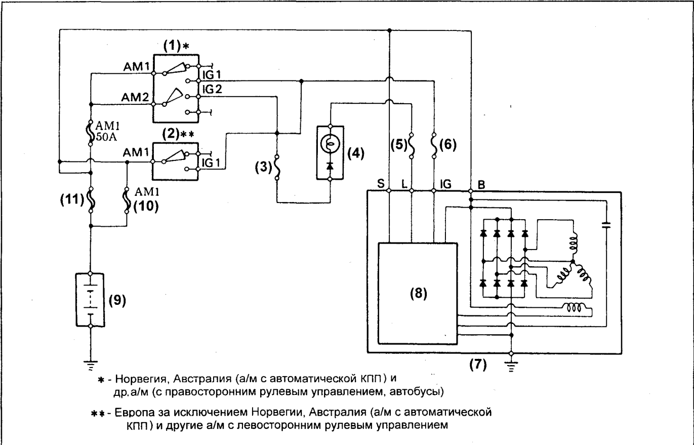
1, 2 - замок зажигания, 3 - предохранитель "IGN" ("Система зажигания") 7,5 А, 4 - контрольная лампа разряда аккумуляторной батареи, 5 - предохранитель "CHG" 7,5 А ("Система зарядки"), 6 - предохранитель "ENGINE" 7,5 А (цепь двигателя), 7 - генератор, 8 - электронный регулятор напряжения, 9 - аккумулятор, 10 - плавкая вставка.
