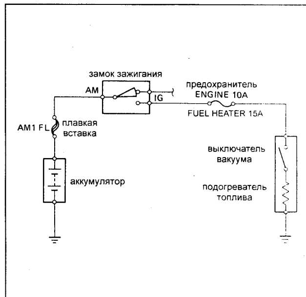
Схема системы подогрева топлива (Land Cruiser Prado 70).
