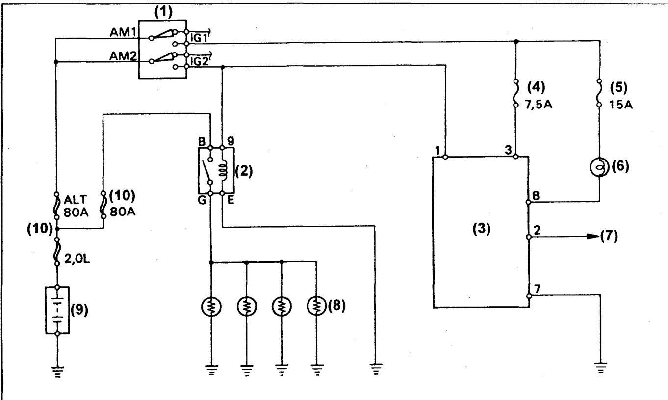
Автомобили HiLux. 1 - замок зажигания, 2 - реле свечей накаливания, 3 - таймер системы управления свечами накаливания, 4, 5 - предохранитель, 6 - контрольная лампа свечей накаливания, 7 - к контрольной лампе разряда аккумулятора, 8 - свечи накаливания, 9 - аккумуляторная батарея, 10 - плавкая вставка.
