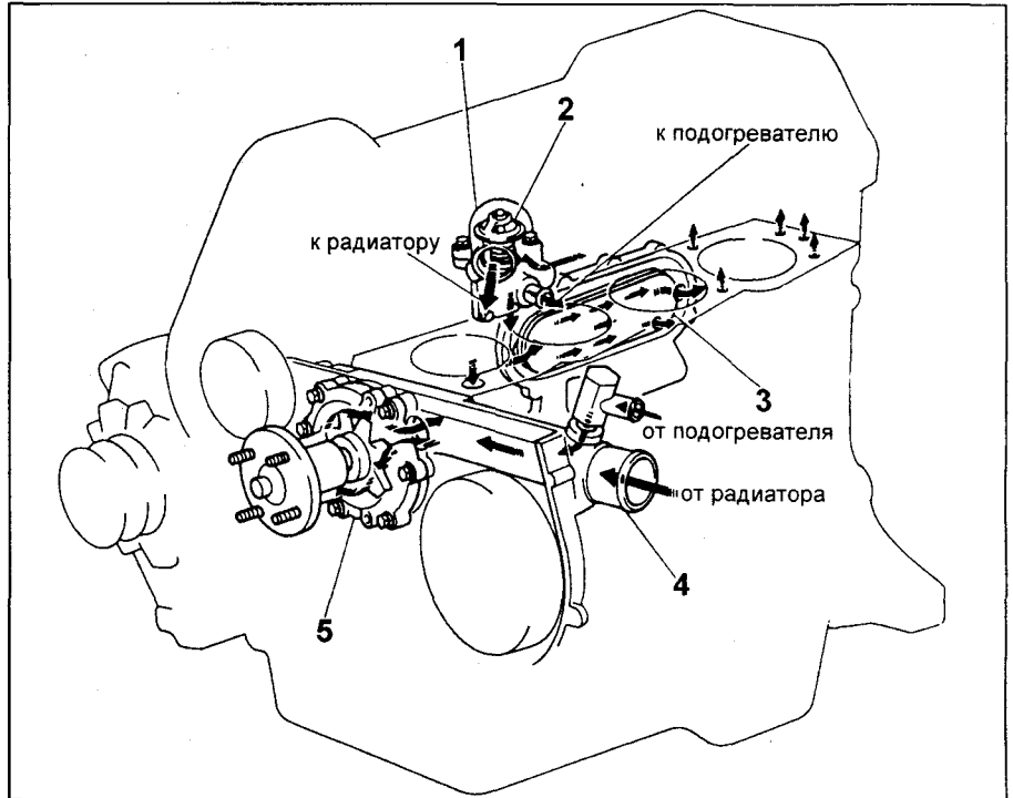
Система охлаждения (двигатель серии L). 1 - корпус термостата, 2 - термостат, 3 - водомасляный радиатор, 4 - патрубок, 5 - насос охлаждающей жидкости.
