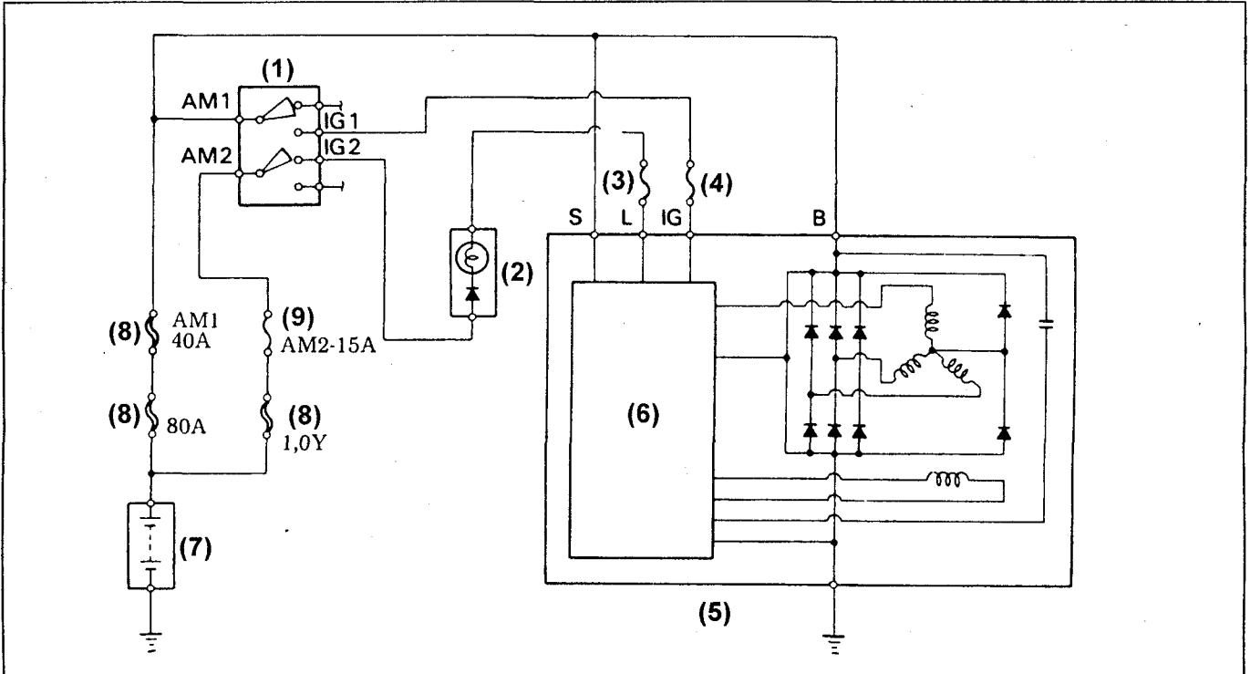
1 - замок зажигания, 2 - контрольная лампа разряда аккумуляторной батареи, 3 - предохранитель "CHG" 7,5 А ("Система зарядки"), 4 - предохранитель "ENGINE" 7,5 А (цепь двигателя), 5 - генератор, 6 - электронный регулятор напряжения, 7 - аккумулятор, 8 - плавкая вставка, 9 - предохранитель.
