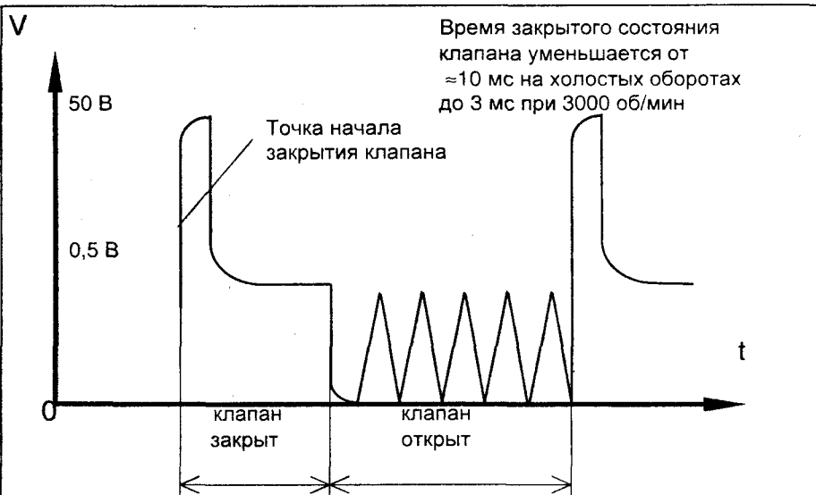
Рис. 5. Диаграмма изменения напряжения, подводимого на обмотку электромагнитного перепускного клапана.
