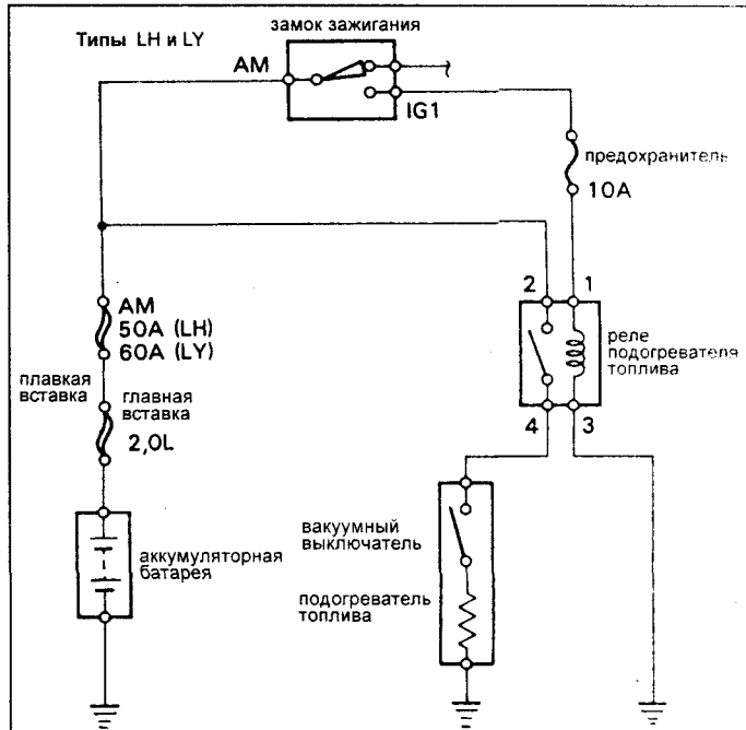
Схема системы подогрева топлива (DYNA).
