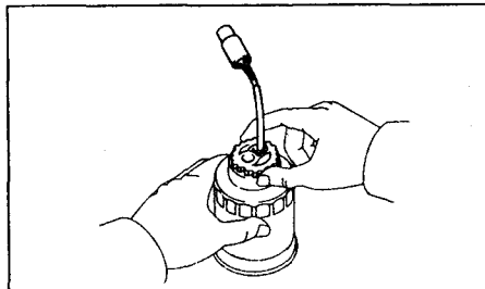
Г. Установите топливный фильтр.
