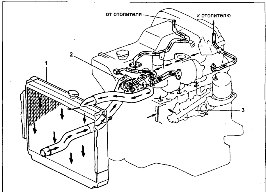
Система охлаждения (двигатель 1KZ-T). 1 - радиатор, 2 - термостат, 3 - маслоохладитель.
