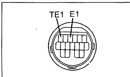
Разъем TDCL (шины данных фирмы Toyota).
