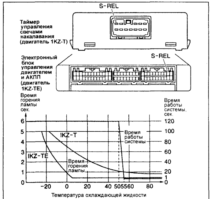
Проверка времени горения контрольной лампы и работы системы - Land Cruiser Prado (KZJ90, 95) двигатель 1KZ-T и 1KZ-TE.
