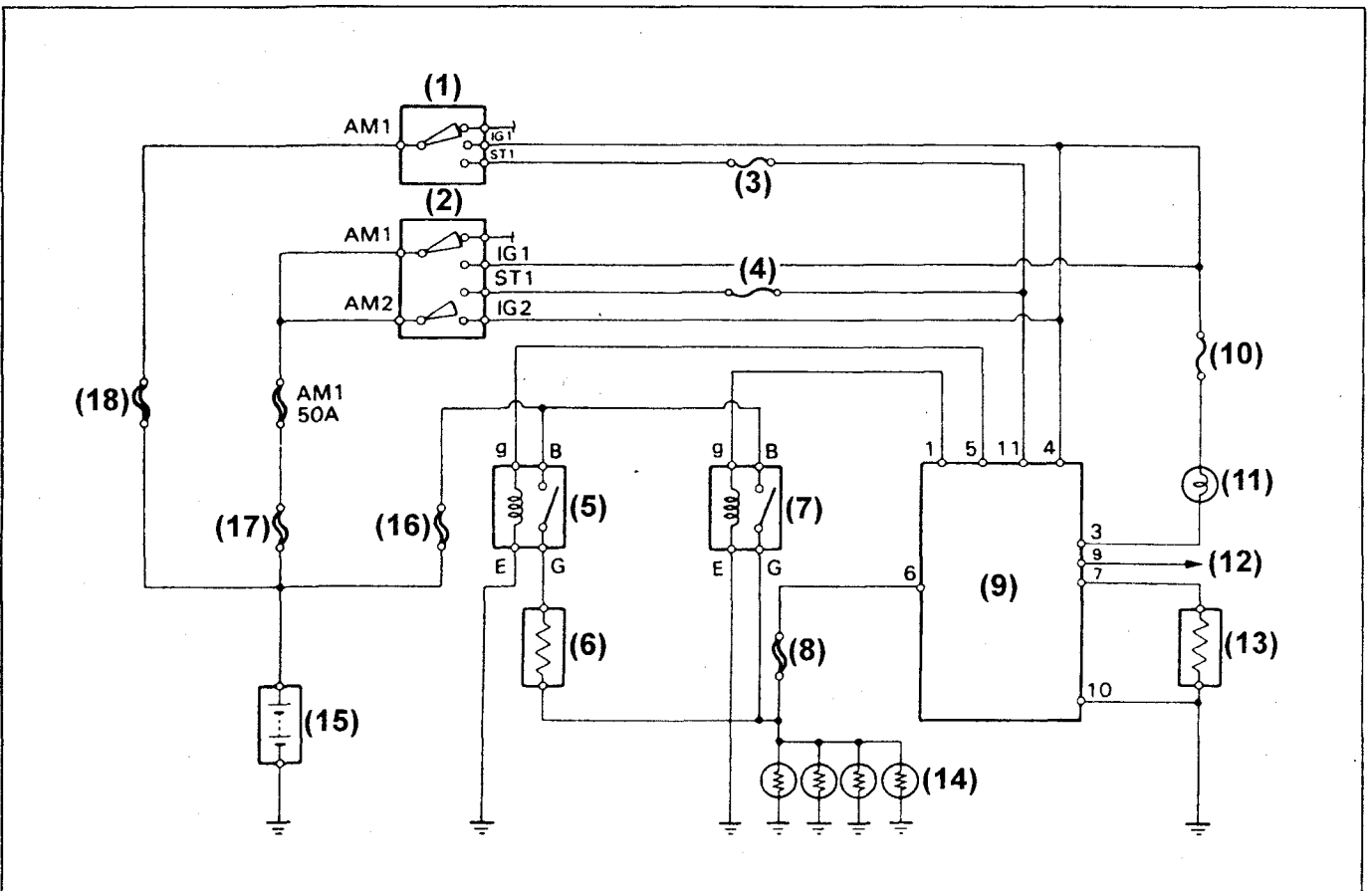
Автомобили НiАсе (Европа). 1 и 2 - замок зажигания (кроме Норвегии и для Норвегии соответственно), 3, 4 - предохранитель стартера 7,5 А, 5 - реле № 2 свечи накаливания, 6 - резистор свечи накаливания, 7 - реле № 1 свечи накаливания, 8 - плавкая вставка 0,3 P, 9 - таймер системы облегчения пуска, 10 - предохранитель, 11 - контрольная лампа свечей накаливания, 12 - к контрольной лампе разряда аккумулятора, 13 - датчик температуры охлаждающей жидкости, 14 - свечи накаливания, 15 - аккумулятор, 16 - плавкая вставка свечи накаливания 80 А, 17 - плавкая вставка генератора 100 А, 18 - плавкая вставка (80 А для типа LY, 60 А для типа LH).
